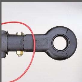
DIN-sjorrog voor in hoogte verstelbare trekdissel
